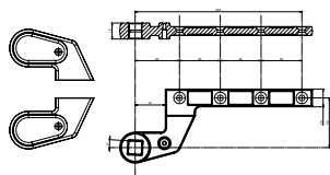
AC583 Braccio universale reversibile con forature
