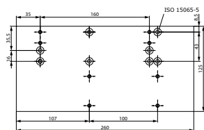
Kit Tandem con piastra di montaggio e perno millerighe
