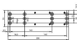
Piastra di montaggio A161
