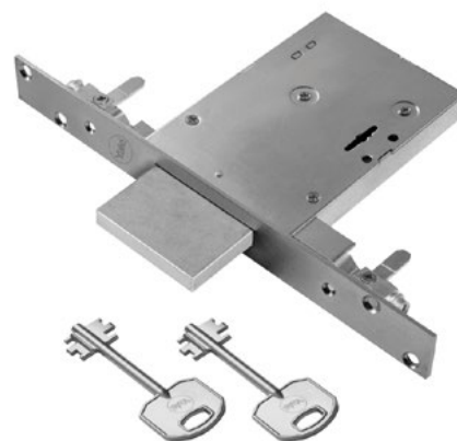
Foto e disegno modello a 3 punti di chiusura
