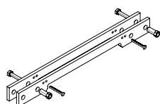
Piastra di montaggio per inferriata
